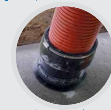
Piquage à 90° (manchon souple) DN 100, 160, 200 & 250mm Collecteur à paroi épaisse 21 - 150mm DN 250 - 1500mm
