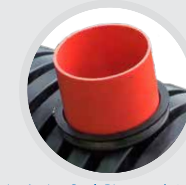
Joint Insitu-Seal, Piquage à 90° DN 110 & 160mm Collecteur annelé DN 200 - 315mm
